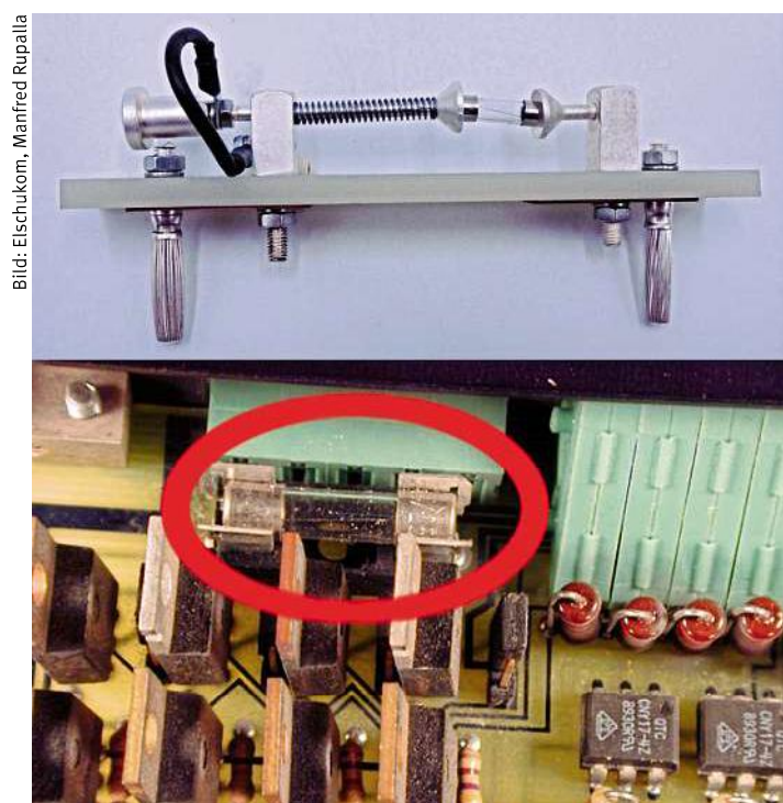
Bild 1: Vergleich einer Sicherung in einem Prüfhalter nach DIN IEC 60127-2 (oben) und mit dem Einsatz in einem Clip-Halter in der Praxis (unten).
